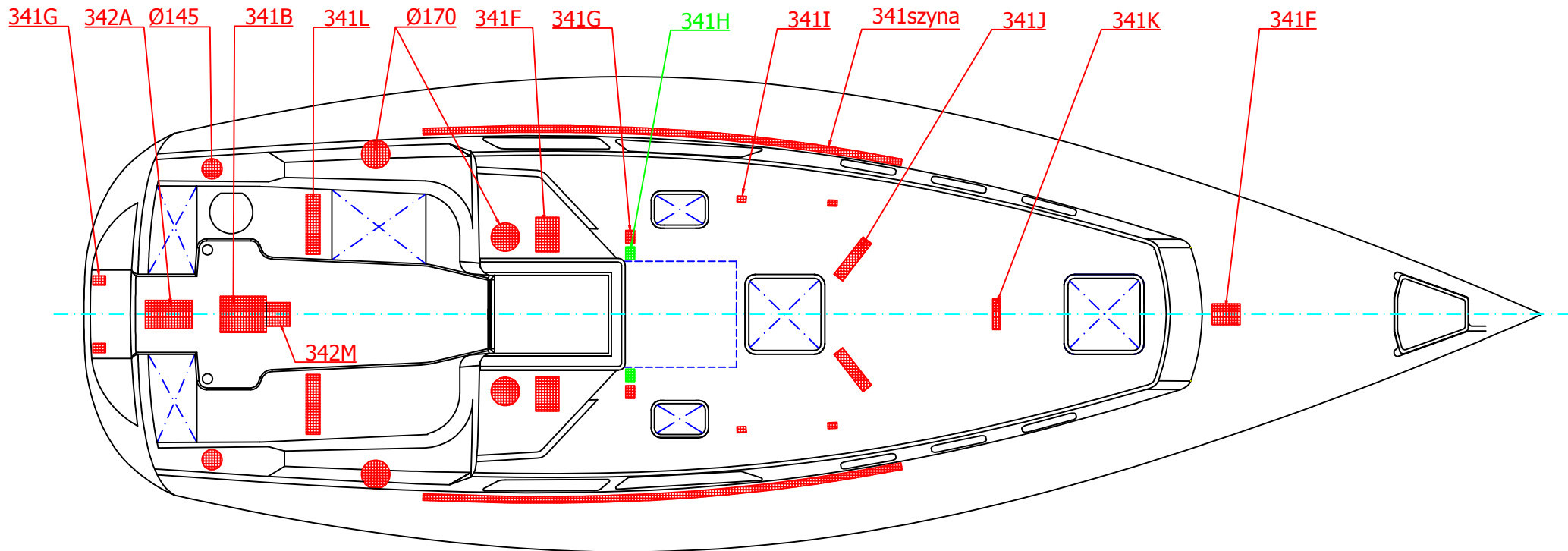
WYKAZ WZMOCNIEŃ METALOWYCH. List of metal reinforcements.
